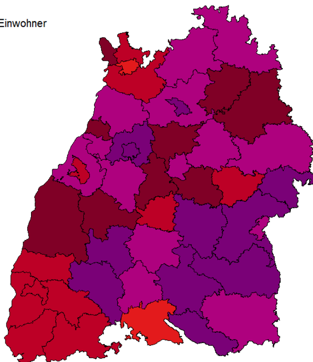
Abbildung 3: 7-Tage-Inzidenz der übermittelten COVID-19-Fälle pro 100.000 Einwohner nach Meldelandkreis, Baden-Württemberg, Stand: 08.11.2021, 16:00 Uhr.
