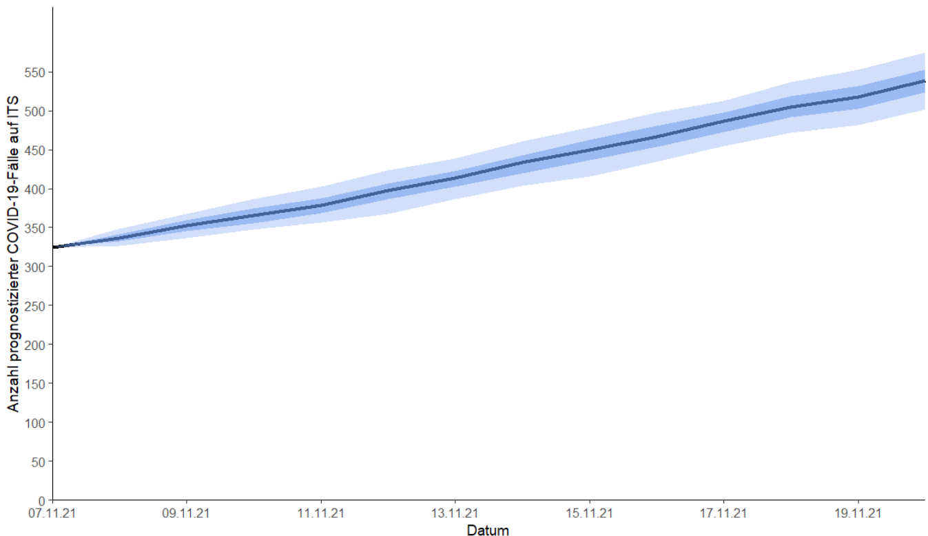
Abbildung 5: Anzahl prognostizierter COVID-19-Fälle auf ITS nach Datum ab dem 07.11.2021 für 14 Tage mit Interquartilsabstand (dunkel) und 95%-Vorhersageintervall (hell), Stand RKI und DIVI-Intensivregister ( www.intensivregister.de ): 08.11.2021, 15:30 Uhr. (Quelle: Berechnungen auf der Basis des Modells des Instituts für Infektionsprävention und Krankenhaushygiene, Universitätsklinikum Freiburg)
