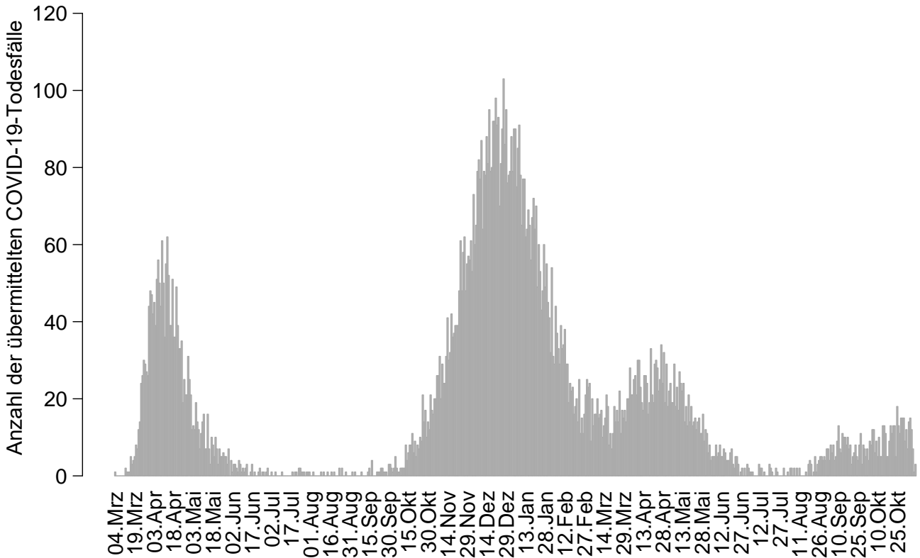
Abbildung 4: Anzahl der übermittelten Fälle, die mit und an COVID-19 verstorben sind, nach Sterbedatum, Baden-Württemberg, Stand: 08.11.2021, 16:00 Uhr.
