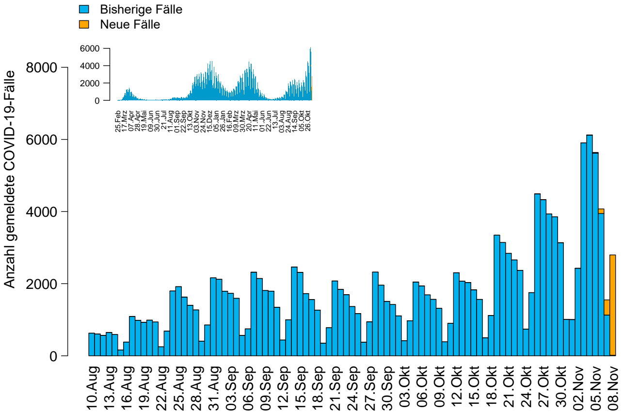
Abbildung 2: Anzahl der übermittelten COVID-19-Fälle nach Meldedatum (blau: bisherige Fälle; gelb: neu übermittelte Fälle), Baden-Württemberg, Stand: 08.11.2021, 16:00 Uhr.
